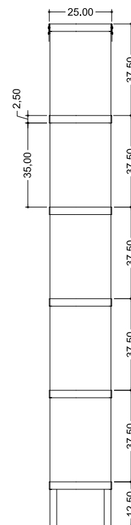
SECÇÃO LATERAL
