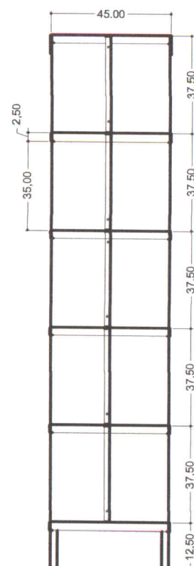
SECÇÃO LATERAL
