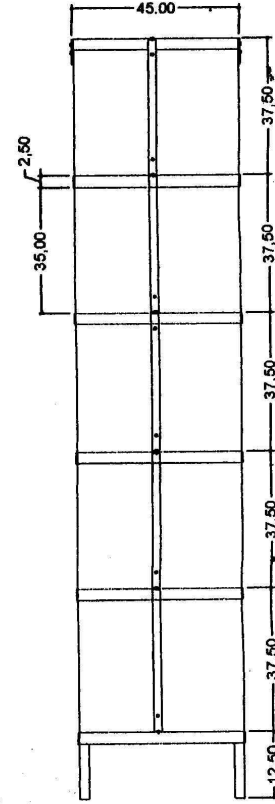
SECÇÃO LATERAL
